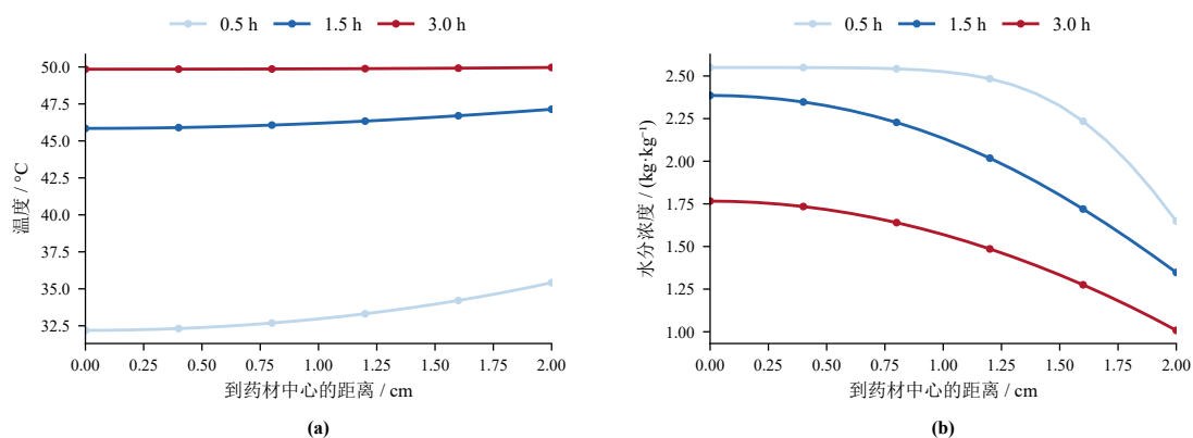
图 5 问题二变物性温度与水分剖面
