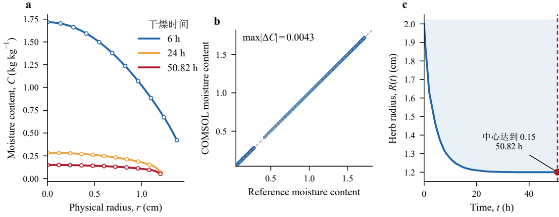
COMSOL 物理场剖面、独立数值校核与收缩历程
