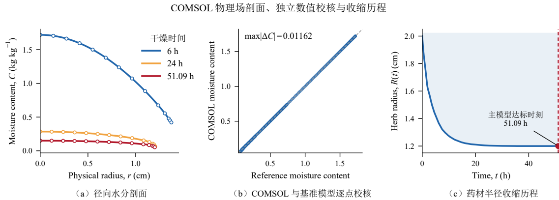
图 13 COMSOL 有限元剖面、原有限体积结果校核与半径收缩历程
