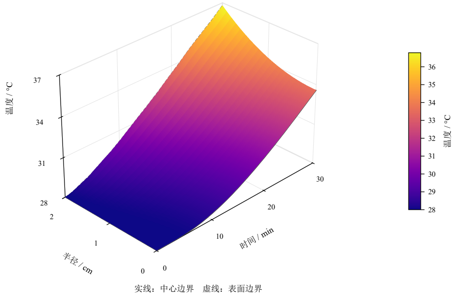
图 4 问题一预热温度的三维时空曲面（0–30 min）
