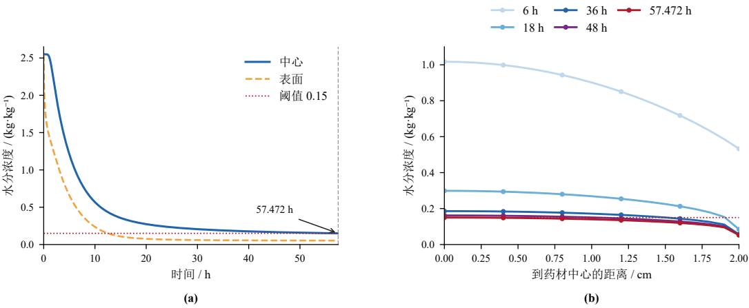
图 8 问题三阈值首达过程与径向分布
