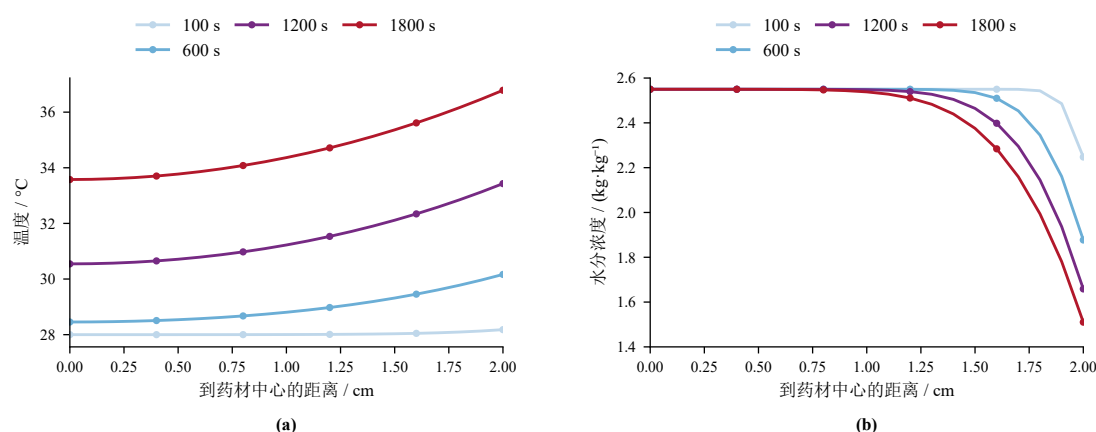
图 3 问题一温度与水分径向剖面
