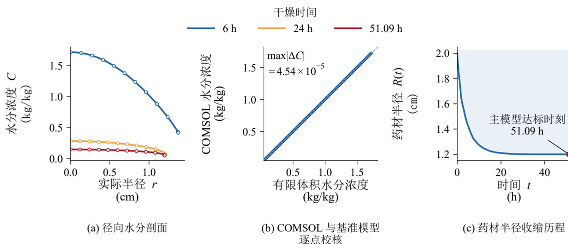
图 13 加密 COMSOL 有限元与有限体积解的剖面对照及半径收缩历程
