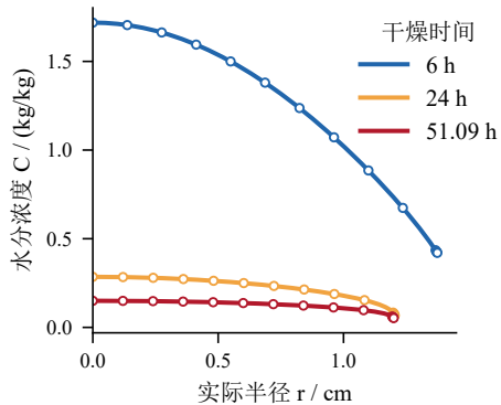
(a) 径向水分剖面
