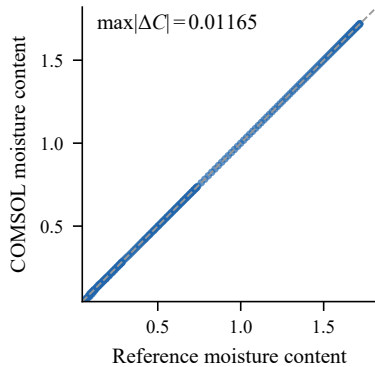
(b) COMSOL 与基准模型逐点校核
