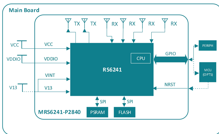
图 2-1 MRS6241-P2840-M81 系统应用框图
