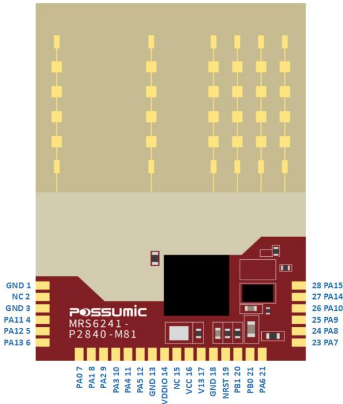
图 3-1 PIN 脚排布
