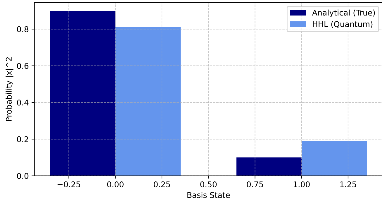
2x2 Integer Eigenvalues
