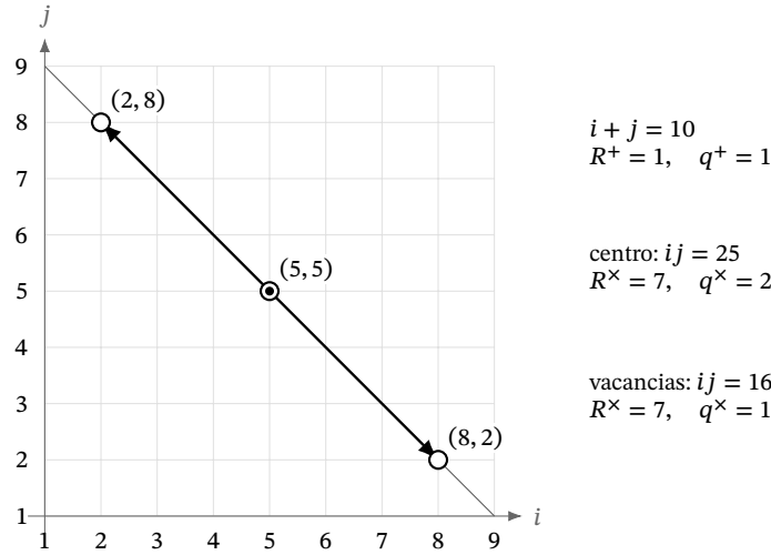
Figura 8: Centro electrónico y vacancias conjugadas en la coordenatización APP. La diagonal es la fibra aditiva \mathcal{F}_{10} ; el centro es el punto fijo de (i, j) \mapsto (10 - i, 10 - j) . Los dos desplazamientos de módulo 3 conservan la suma y el residuo producto y reducen en una unidad el cociente multiplicativo. Las flechas representan las deformaciones sobre la fibra.
