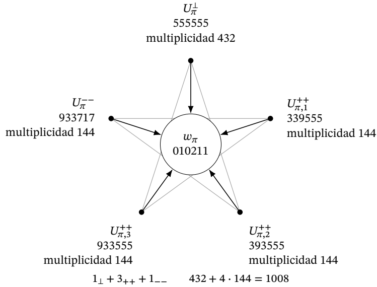
Figura 11: Las cinco regiones de \pi en disposición pentádica. Cada posición conserva su firma multiplicativa y su multiplicidad; las flechas radiales representan la proyección común \Psi(U) = 010211 . El contorno estrellado organiza las cinco posiciones de la coordenatización. Su realización en las cinco octadas de Witt se efectúa mediante el alineamiento regional y la descomposición 4 + 1 del texto.
