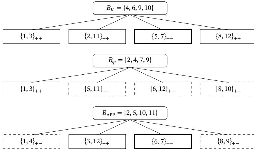
Figura 10: Comparación de las tres estrellas. Cada conexión representa la unión de la cuaterna superior con un par; las doce hexadas completas figuran en la tabla 12. El contorno grueso señala los pares negativos y el discontinuo los mixtos. Las conexiones representan incidencia.
