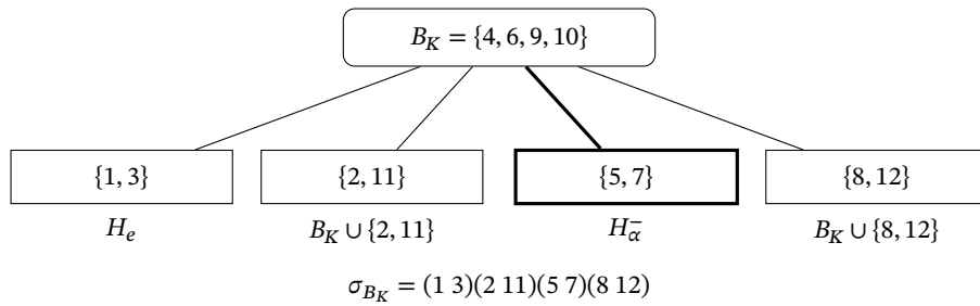
Figura 9: La estrella concreta de la bandera dodecafásica. Cada línea indica la unión de la cuaterna central con el par de su extremo; la línea gruesa señala la hexada seleccionada también por los signos anteriores al acarreo de \alpha . Los cuatro pares agotan las ocho posiciones exteriores.
