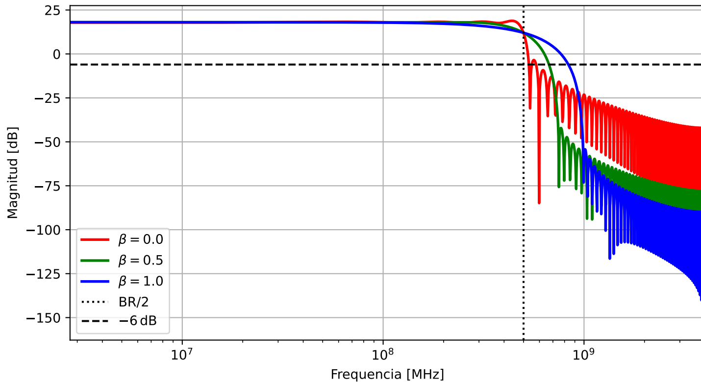
Respuesta en Frecuencia (Punto Flotante). BR = 1 GBd. OS = 8
