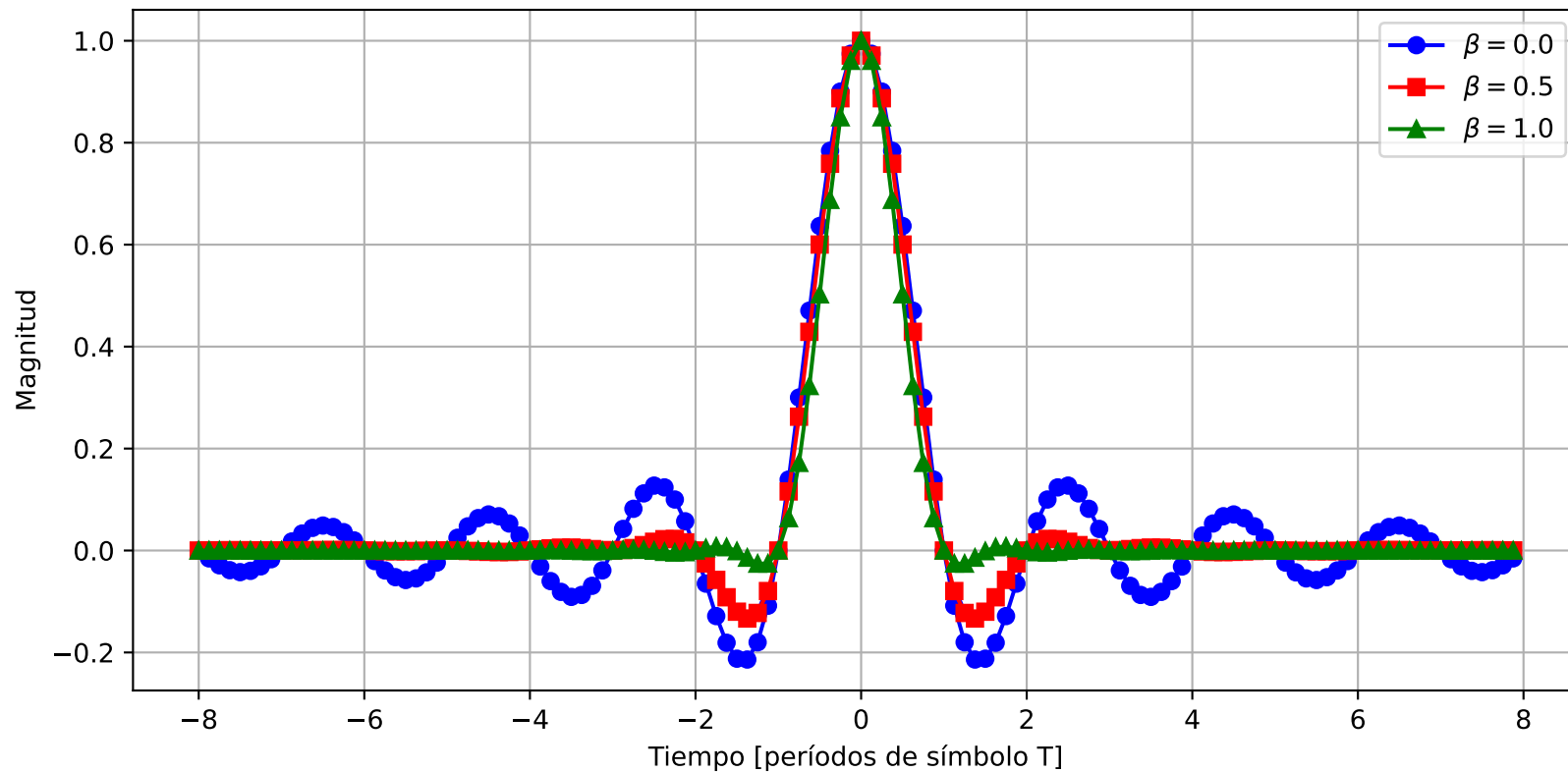
Respuesta al Impulso (Punto Flotante). BR = 1 GBd. OS = 8
