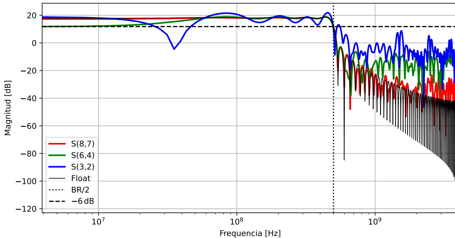
Respuesta en Frecuencia. \beta = 0
