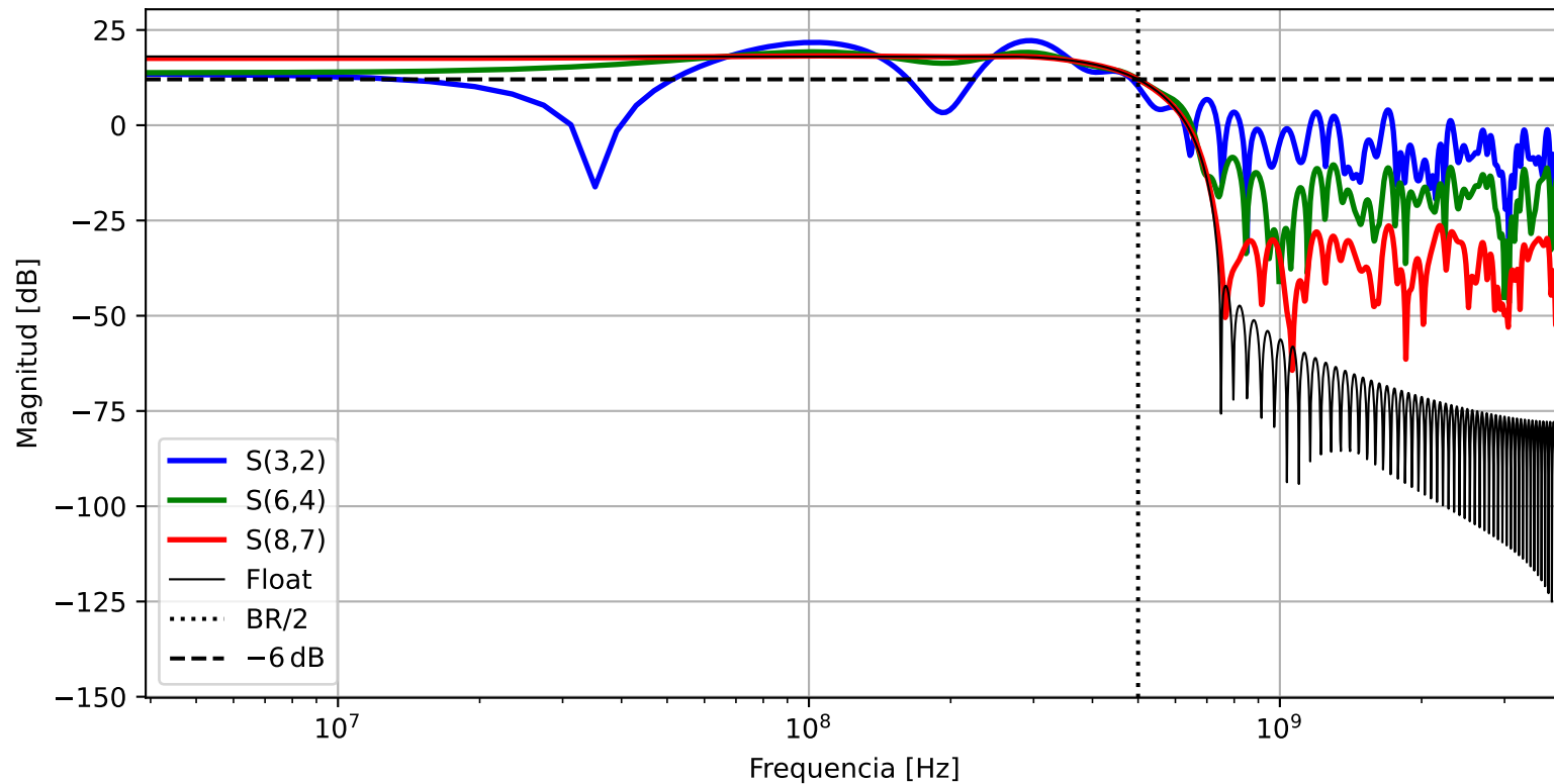
Respuesta en Frecuencia. \beta = 0.5
