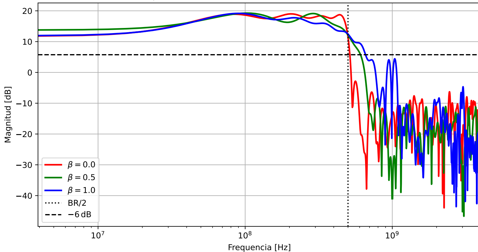
Respuesta en Frecuencia. Formato: S(6,4) Truncado
