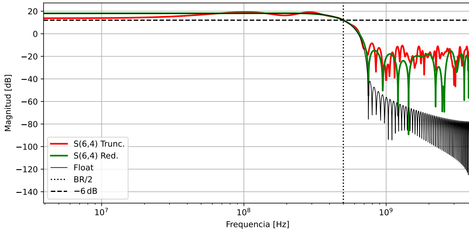
Respuesta en Frecuencia. \beta = 0.5 . Formato: S(6,4)
