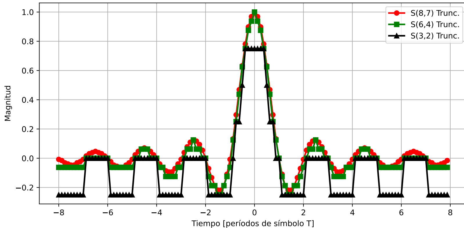
Respuesta al Impulso. \beta = 0
