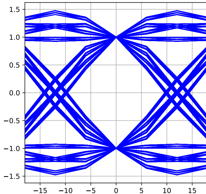
Diagrama de ojo (Q)
