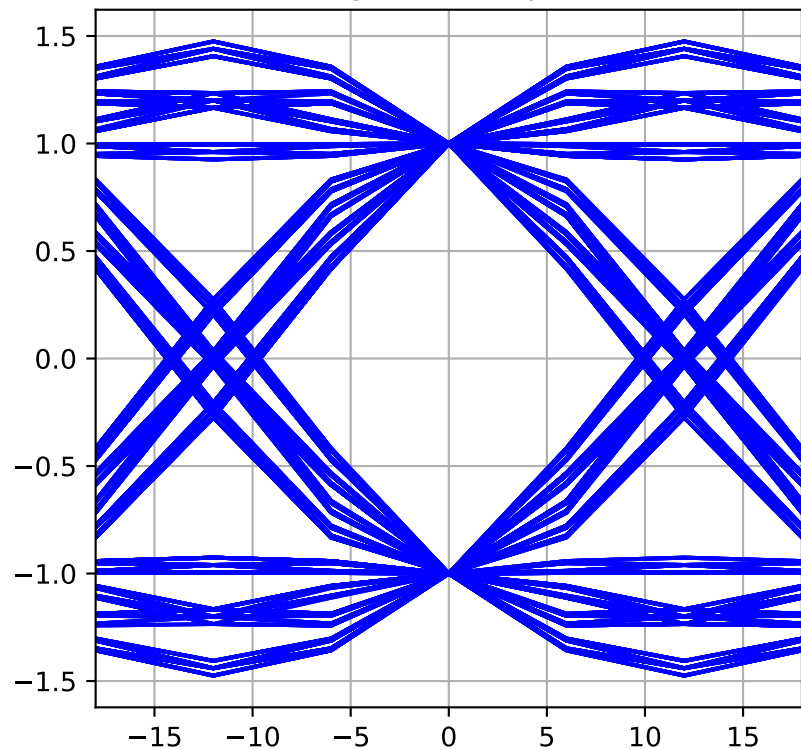
Diagrama de ojo (I)
