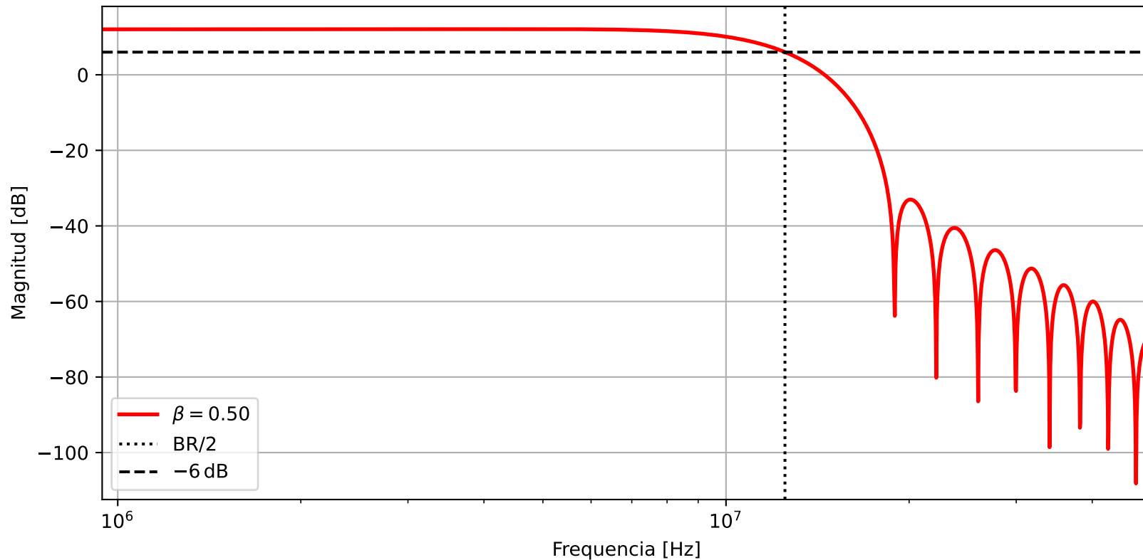
Respuesta en Frecuencia. BR = 25.0 MBd. OS = 4
