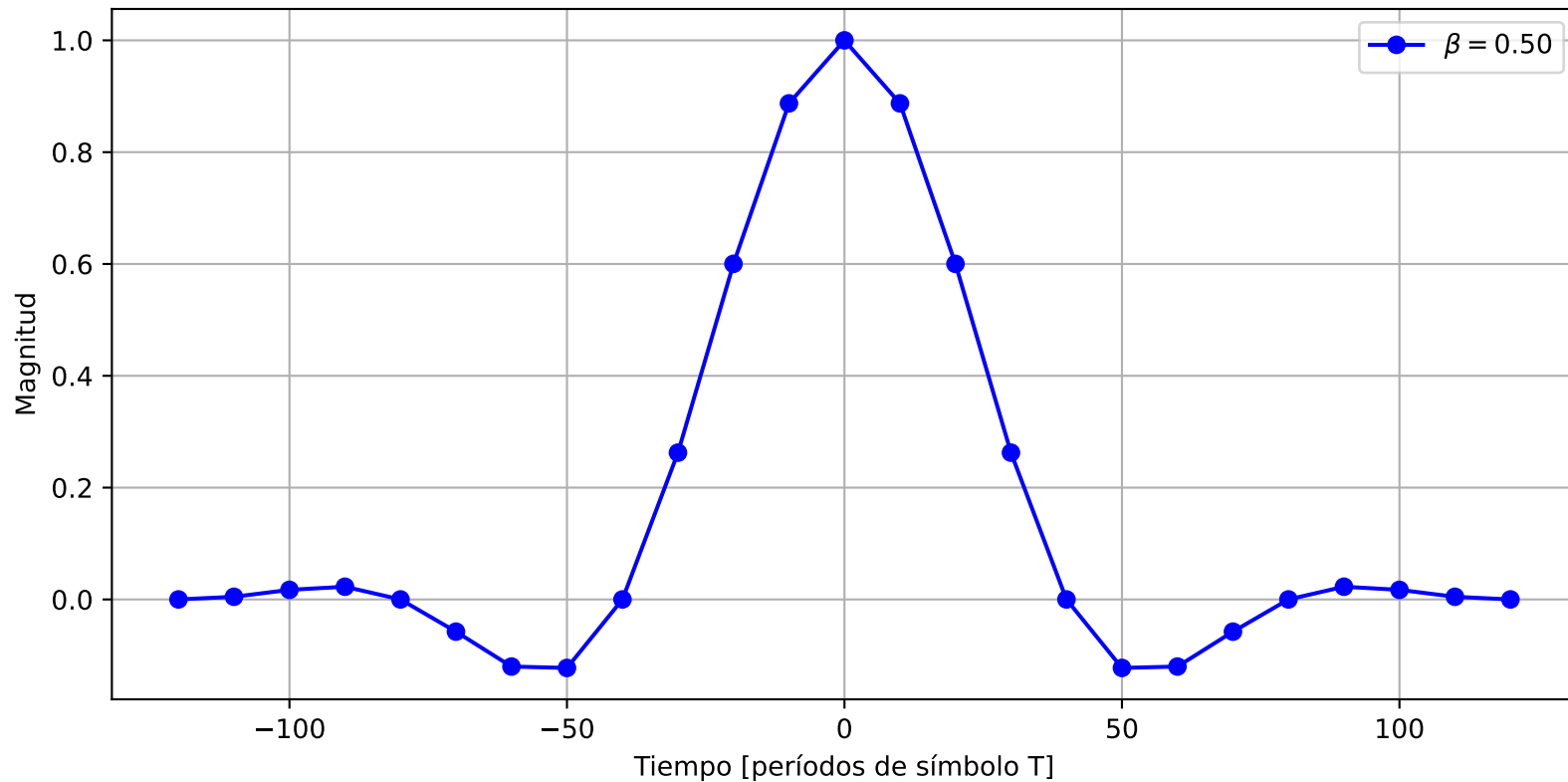
Respuesta al Impulso. BR = 25.0 MBd. OS = 4
