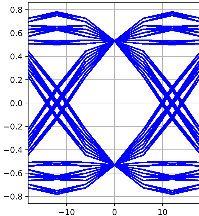
Diagrama de ojo (Q)
