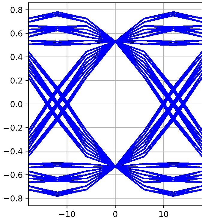
Diagrama de ojo (I)
