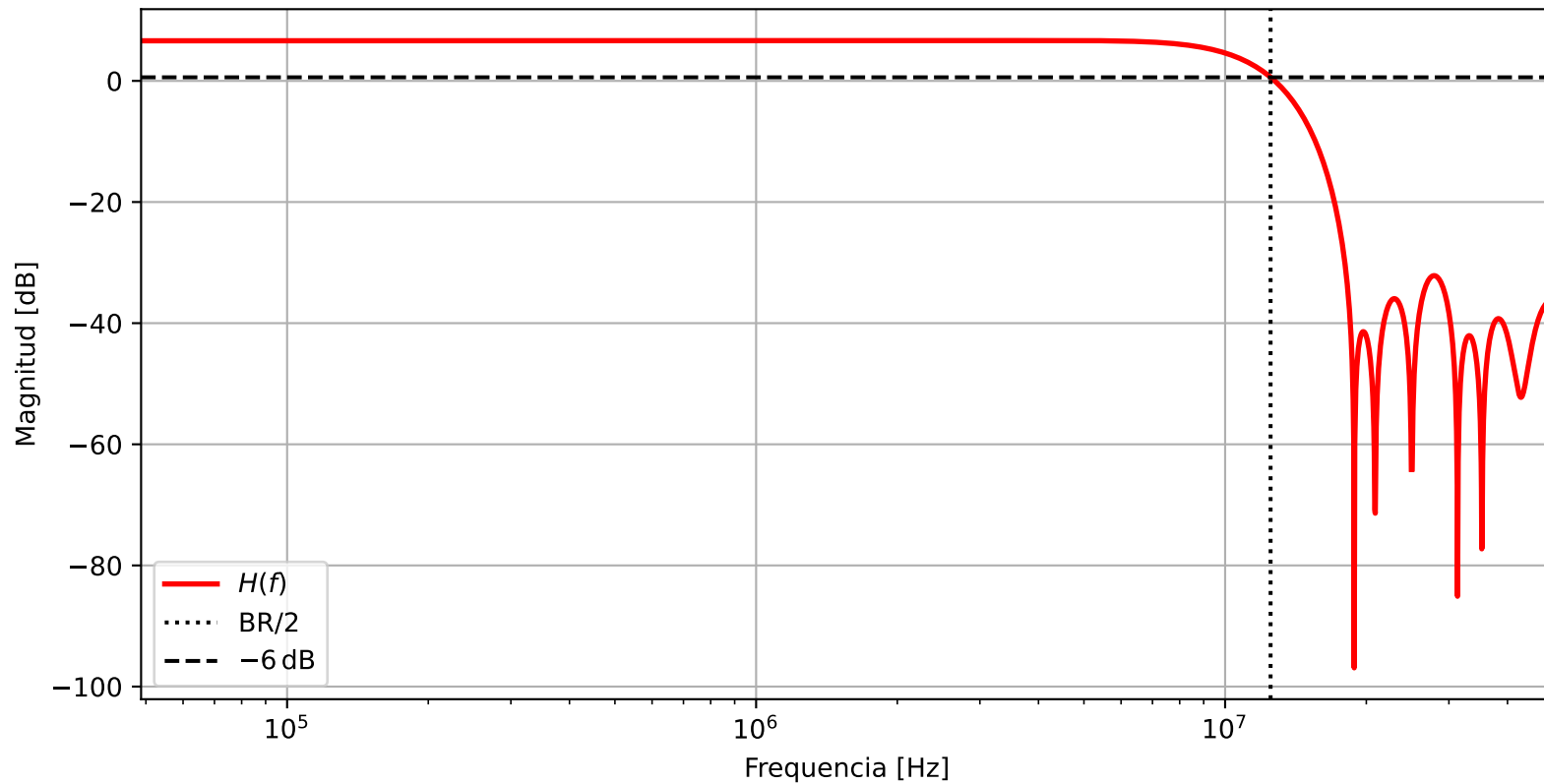
Respuesta en Frecuencia. BR = 25 MBd. OS = 4
