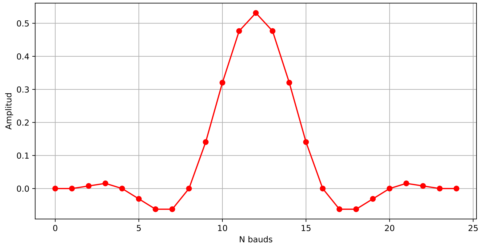
Respuesta al Impulso. OS = 4
