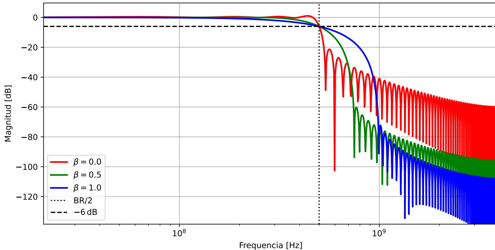
Respuesta en Frecuencia (Punto Flotante). BR = 1 GBd. OS = 8
