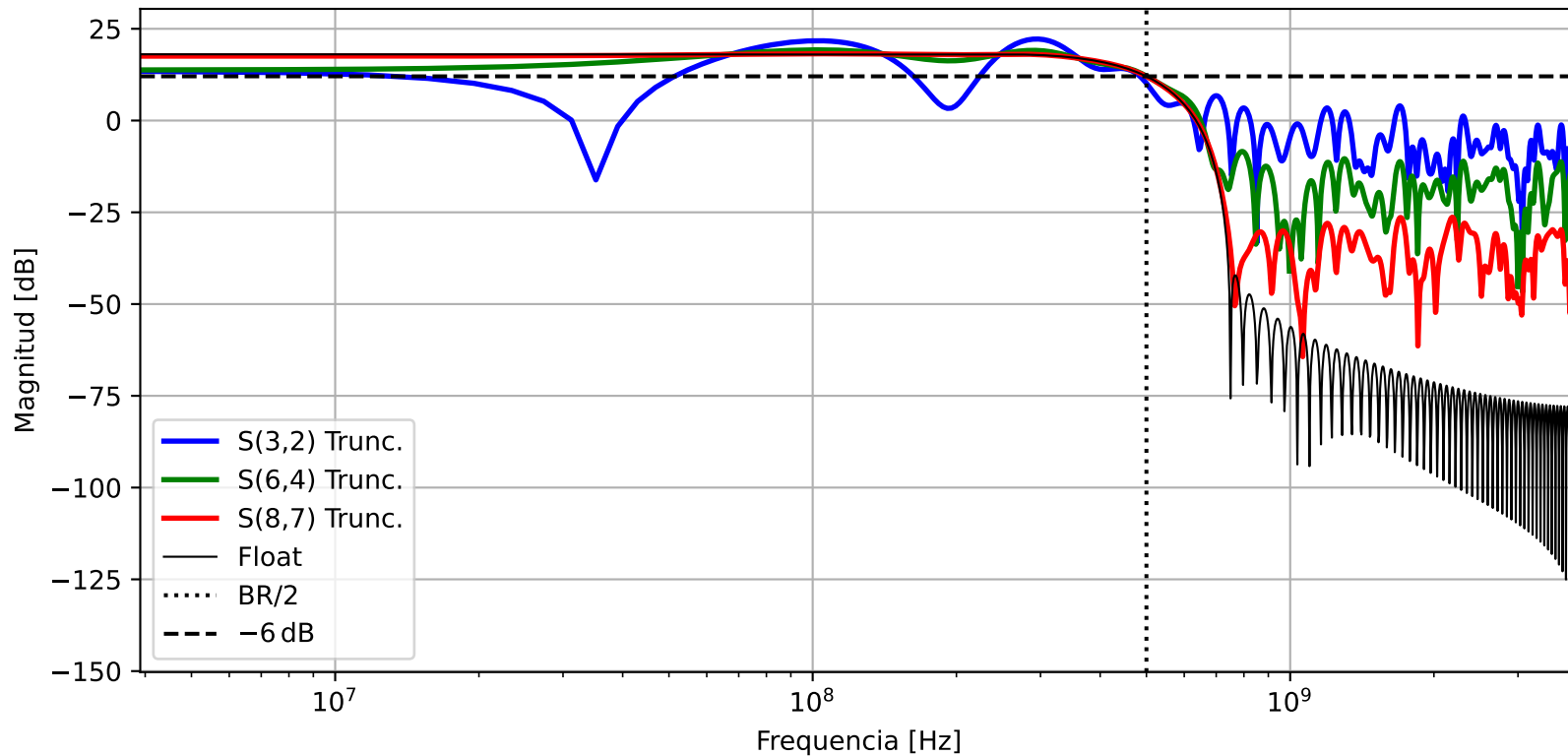
Respuesta en Frecuencia. \beta = 0.5
