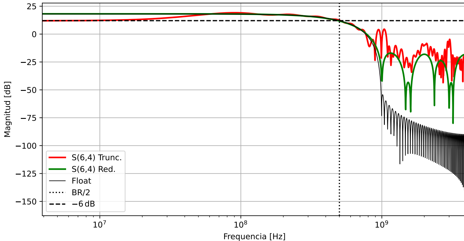
Respuesta en Frecuencia. \beta = 1 . Formato: S(6,4)
