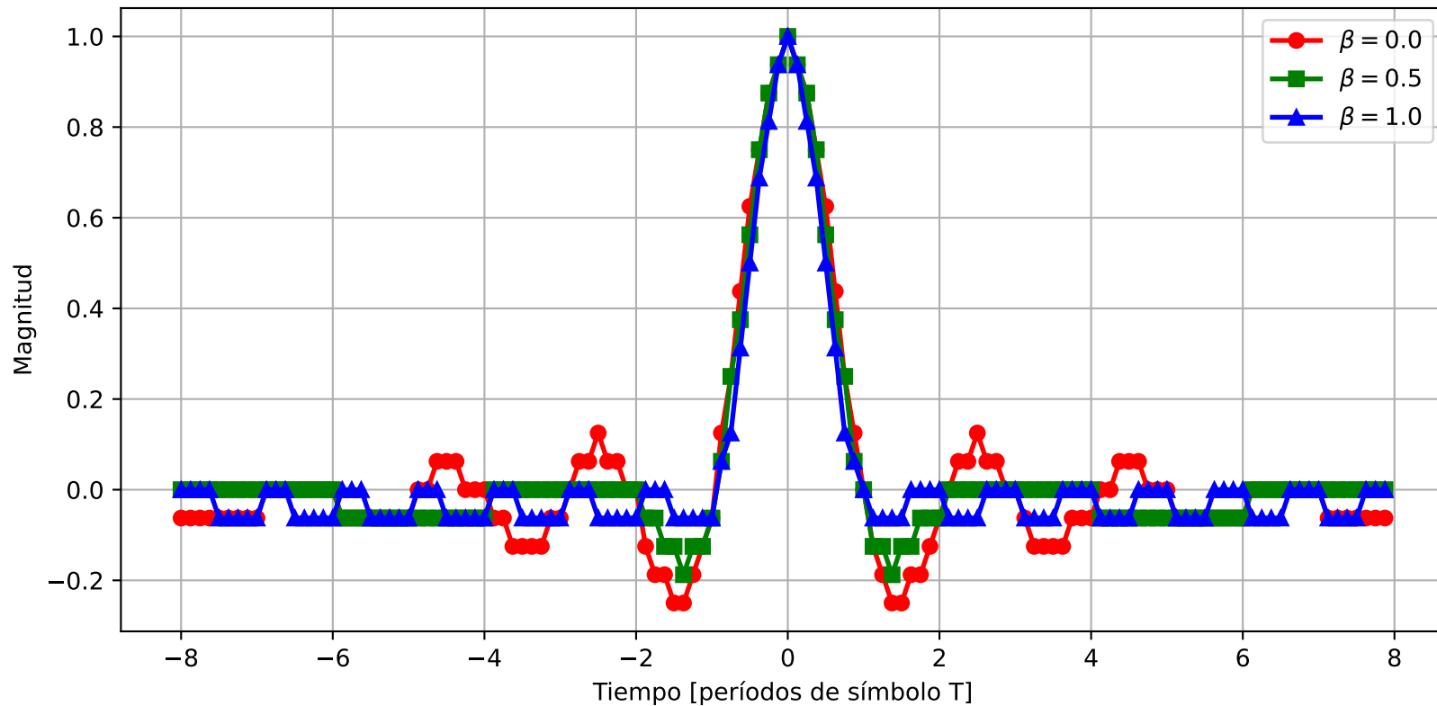
Respuesta al Impulso. Formato: S(6,4) Truncado.
