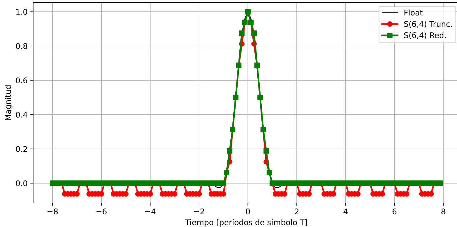
Respuesta al Impulso. \beta = 1 . Formato: S(6,4)
