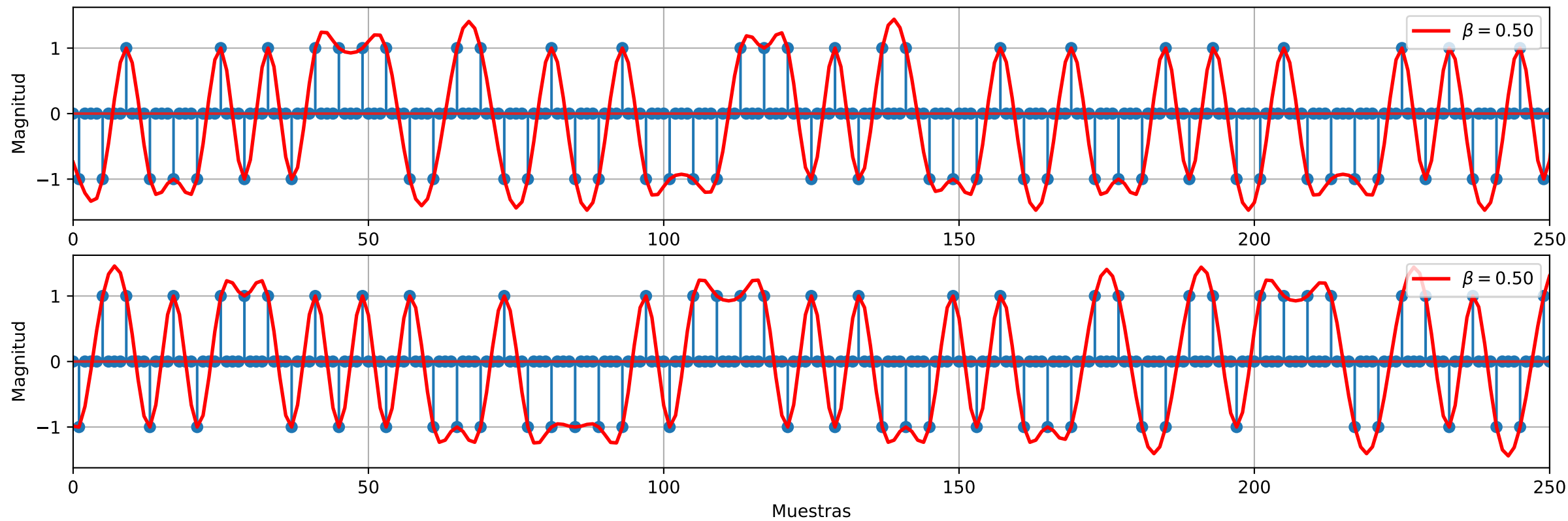
Convolución del RC con símbolos. OS: 4
