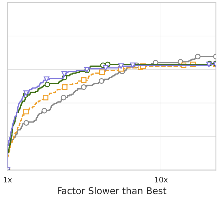
Indexed Cache
