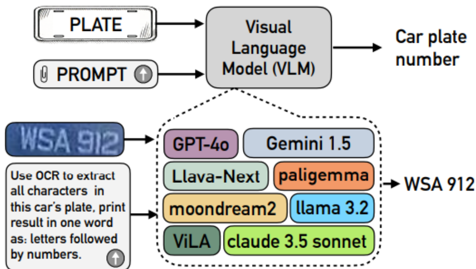
Figura 29: Diagrama de uso de VLMs para reconocer caracteres en matrículas Fuente: https://arxiv.org/pdf/2412.14197
