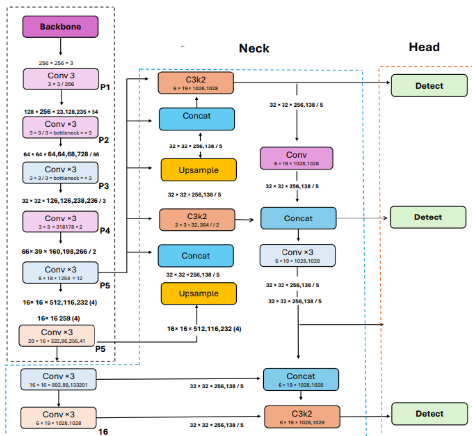
Figura 39: Arquitectura del modelo YOLO26 para detección y segmentación Fuente: https://arxiv.org/pdf/2509.25164
