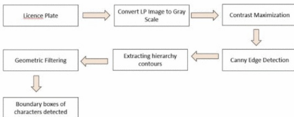
Figura 21: Proceso de flujo de segmentación de matrículas Fuente: https://ieeexplore.ieee.org/document/10183638
