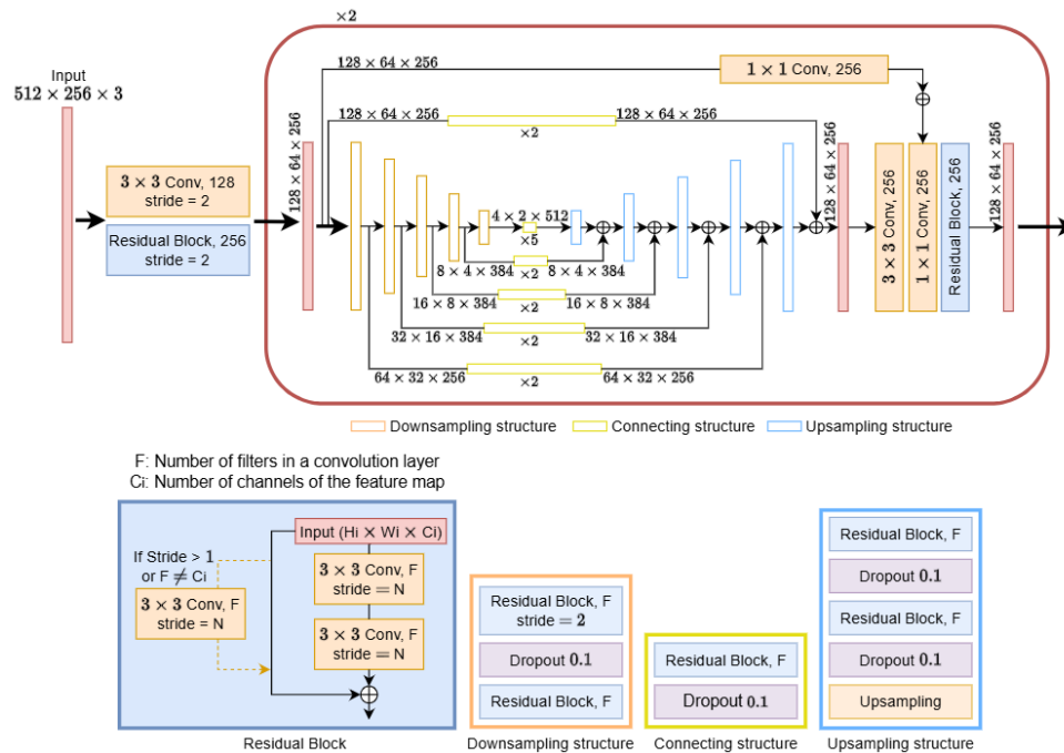
Figura 12: Arquitectura Hourglass
