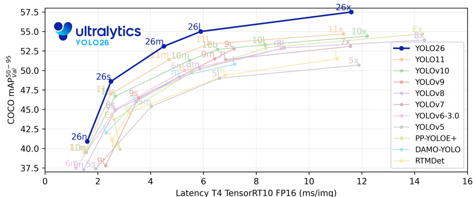
Figura 38: Compensación entre velocidad y precisión entre los distintos modelos YOLO Fuente: https://arxiv.org/pdf/2509.25164
