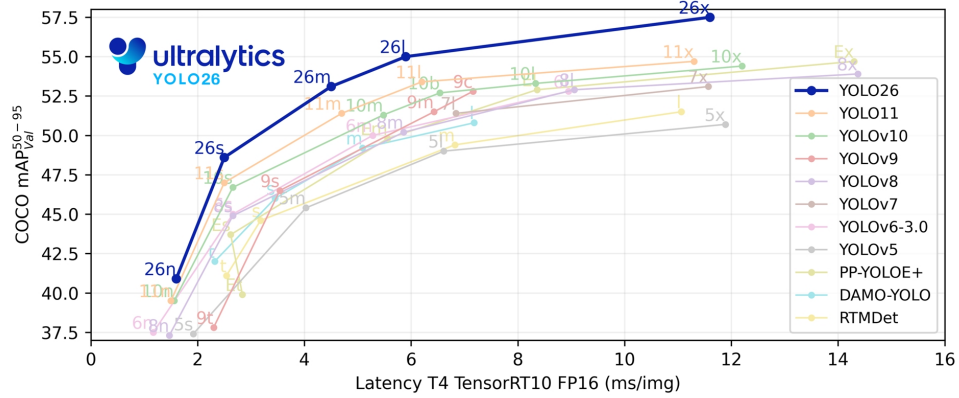
Figura 34: Compensación entre velocidad y precisión entre los distintos modelos YOLO Fuente: https://arxiv.org/pdf/2509.25164
