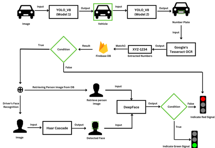
Figura 6: Esquema de flujo de la tarea de detección de vehículos y de matrículas Fuente: https://arxiv.org/pdf/2312.02699
