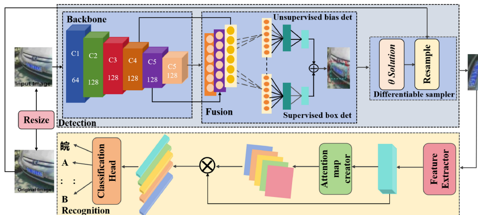
Figura 17: Flujo de un detector de una etapa en reconocimiento de matrículas Fuente: https://www.sciencedirect.com/science/article/pii/S0893608026003047
