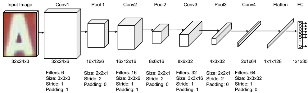
Figura 32: Arquitectura de LeNet-5 modificada
