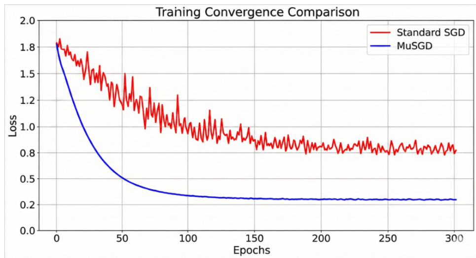
Figura 37: Concepto visual esperado de la optimización dinámica de MuSGD Fuente: https://arxiv.org/html/2601.12882v1
