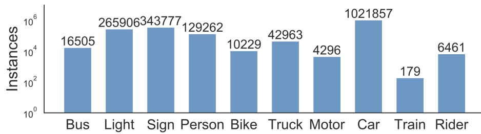
Figura 39: Estadísticas de los diferentes tipos de objetos en el dataset Bdd100k Fuente: https://bair.berkeley.edu/blog/2018/05/30/bdd/
