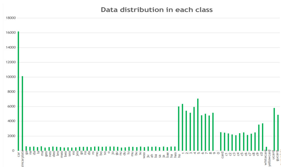
Figura 22: Distribución de clases del conjunto de datos del sistema Shine Fuente: https://arxiv.org/pdf/2302.00837
