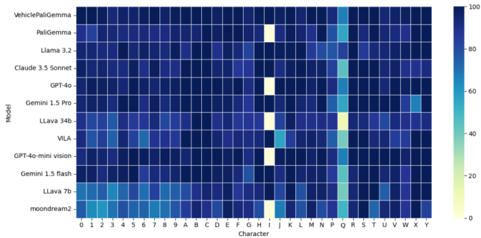
Figura 26: Mapa de calor de la precisión de reconocimiento de caracteres en diferentes VLMs. Fuente: https://arxiv.org/pdf/2412.14197
