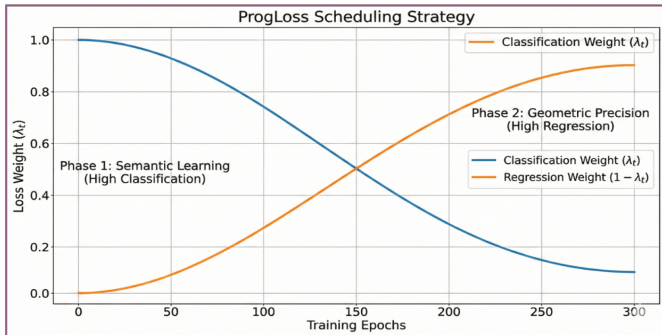
Figura 36: Estrategia de priorización del sistema Progloss Fuente: https://arxiv.org/html/2601.12882v1
