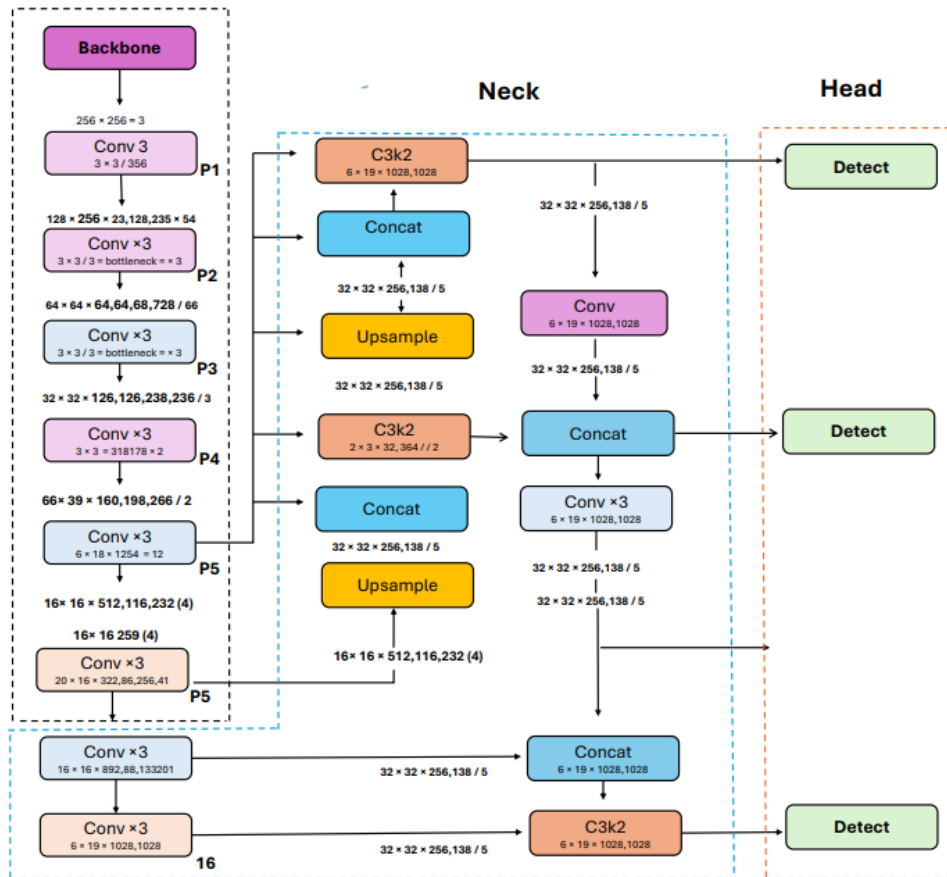
Figura 35: Arquitectura del modelo YOLO26 para detección y segmentación Fuente: https://arxiv.org/pdf/2509.25164
