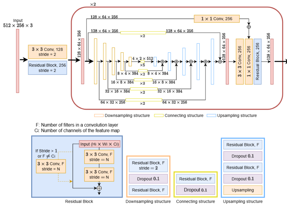
Figura 12: Arquitectura Hourglass
