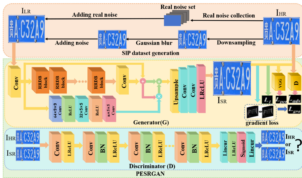
Figura 18: Estructura de un modelo de Deep Learning para el reconocimiento de matrículas Fuente: https://www.sciencedirect.com/science/article/pii/S0893608026003047
