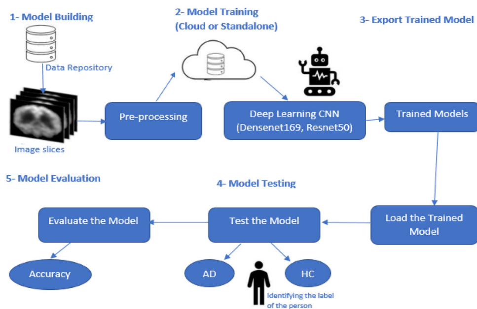
Figura 43: Metodología del diagnóstico y clasificación de Alzheimer con CNNs Fuente: https://peerj.com/articles/cs-1177/
