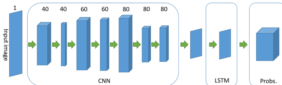
Figura 30: Arquitectura OCR Fuente: https://arxiv.org/pdf/2309.12972
