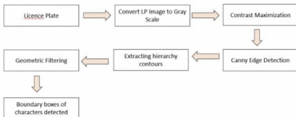
Figura 21: Proceso de flujo de segmentación de matrículas Fuente: https://ieeexplore.ieee.org/document/10183638
