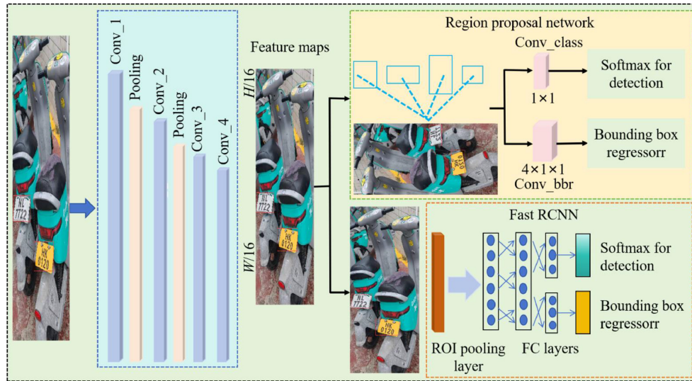
Figura 16: Flujo de un detector de dos etapas en reconocimiento de matrículas Fuente: https://www.sciencedirect.com/science/article/pii/S0893608026003047
