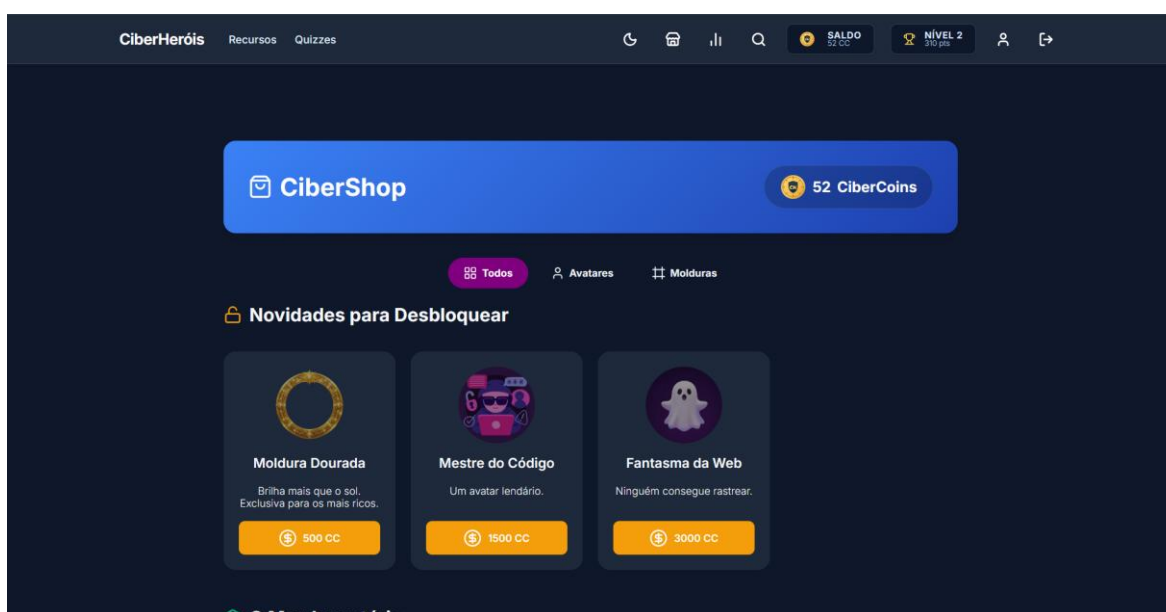
Figura 36 - Página Loja
