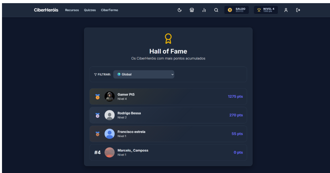
Figura 35 - Página Leaderboard
