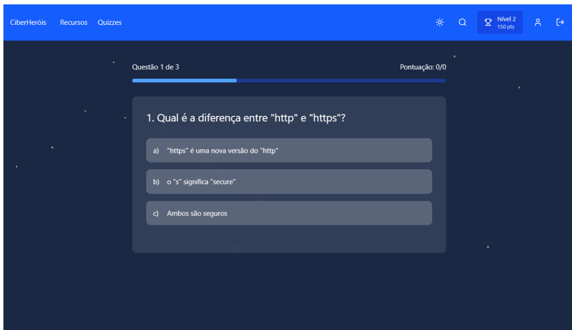
Figura 23 - Mockup Quiz
