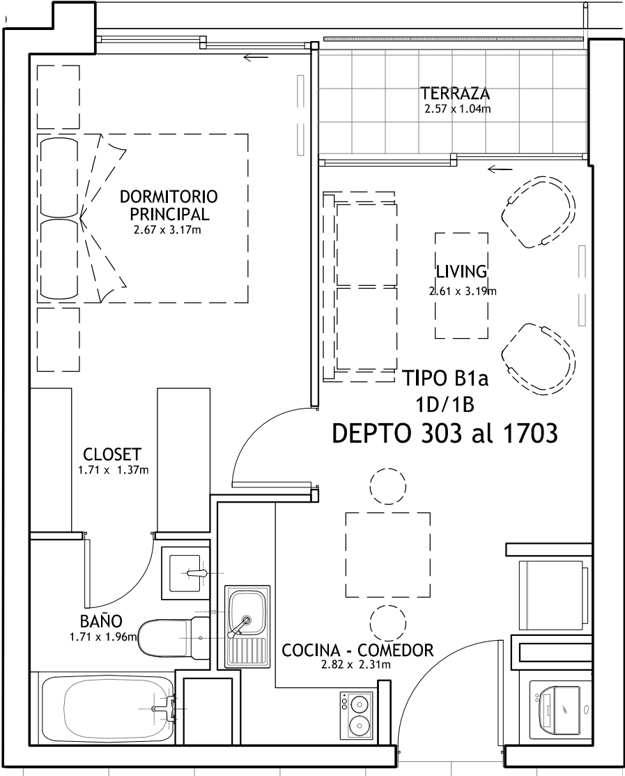
PLANTA PISO 3 al 17 DEPTO N° 303 al 1703
