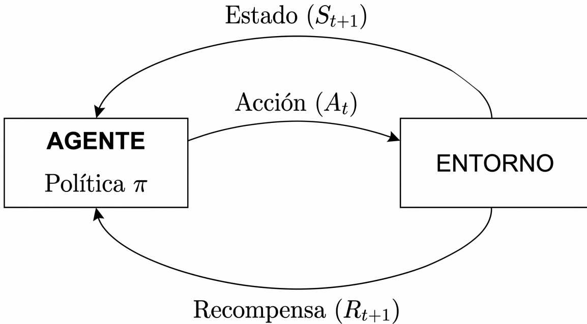
Figure 1.1: Diagrama del proceso de interacción en el aprendizaje por refuerzo.
