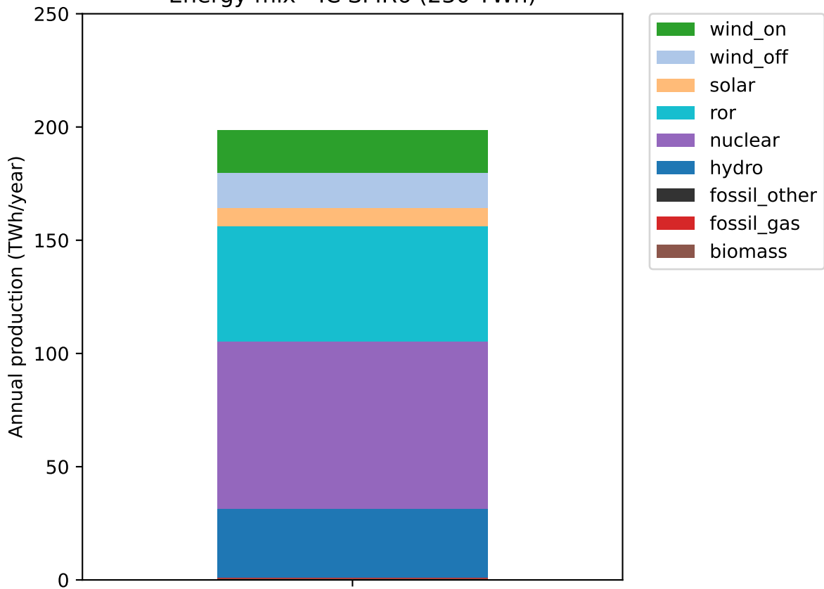
Energy mix - IC SMR6 (230 TWh)
