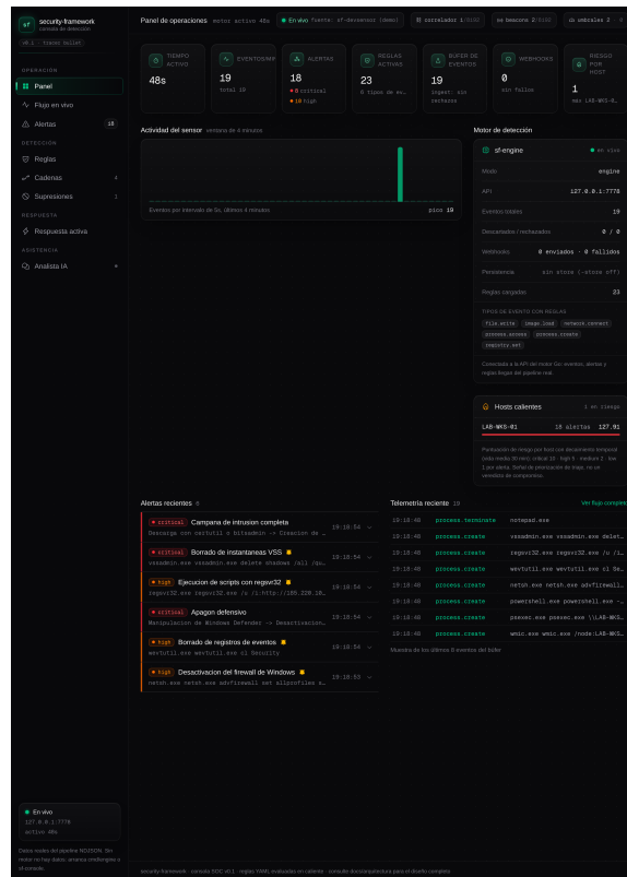
Figura 2. Dashboard de operaciones de la consola: KPIs, actividad del sensor, cola de triaje en vivo y panel de hosts calientes completo. Captura regenerada sobre el árbol vigente (bc53788) con el stack real: la navegación incluye la vista de respuesta activa de la ola C3 de consola y la operabilidad forense posterior — la limitación declarada hasta la v0.6 queda resuelta en esta revisión (recaptura del acta 20h05_B).
