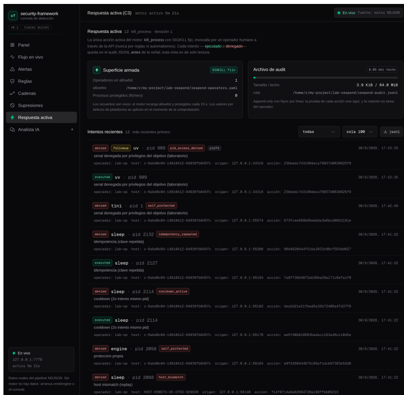
Figura 3. Vista de respuesta activa con la cola «todas» sobre audit real de laboratorio (12 líneas genuinas): el par F1 arriba — executed y su followup denied compartiendo action_id —, badges de seguimiento, etiquetas de mechanism, los 6 códigos de denegación, las tarjetas de superficie armada y de salud del audit, y los tres controles: filtro de clase, ventana de cola 100/500 y export JSONL.
