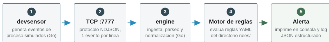
Figura 5. Tracer bullet: pipeline de evento a alerta ejecutable en cualquier plataforma.
