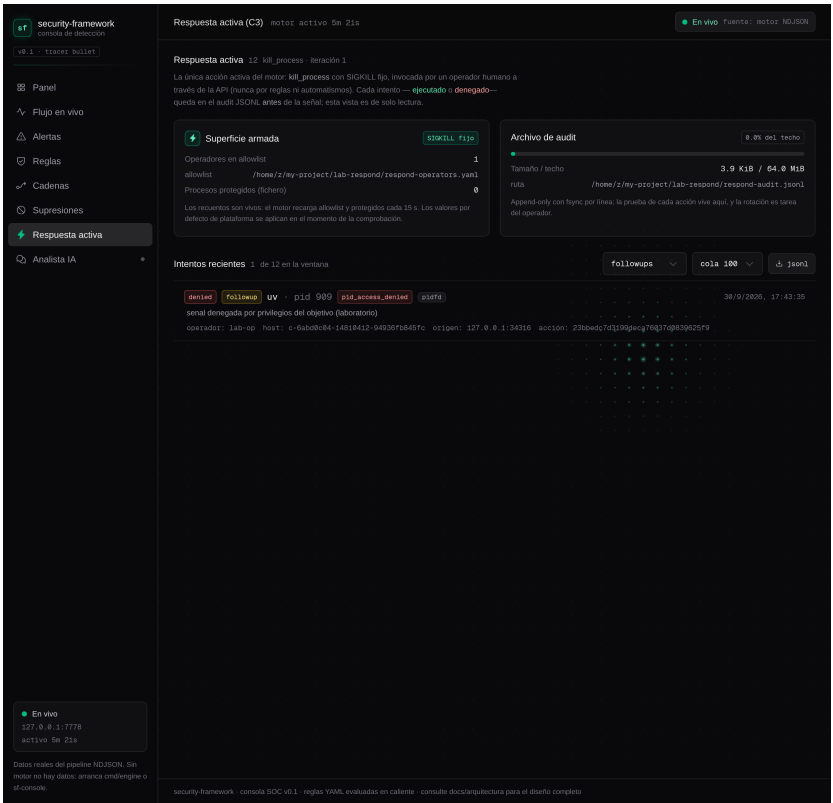
Figura 4. Filtro de clase en «followups»: conteo honesto «1 · de 12 en la ventana» y la única fila followup real (pid_access_denied del par F1) — la toma exacta que el guion de la ronda 19h25 pidió.
