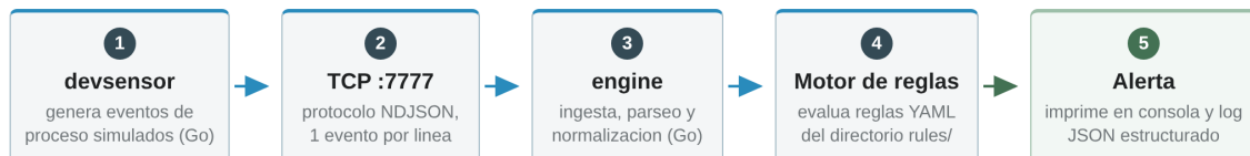
Figura 3. Tracer bullet: pipeline de evento a alerta ejecutable en cualquier plataforma.
