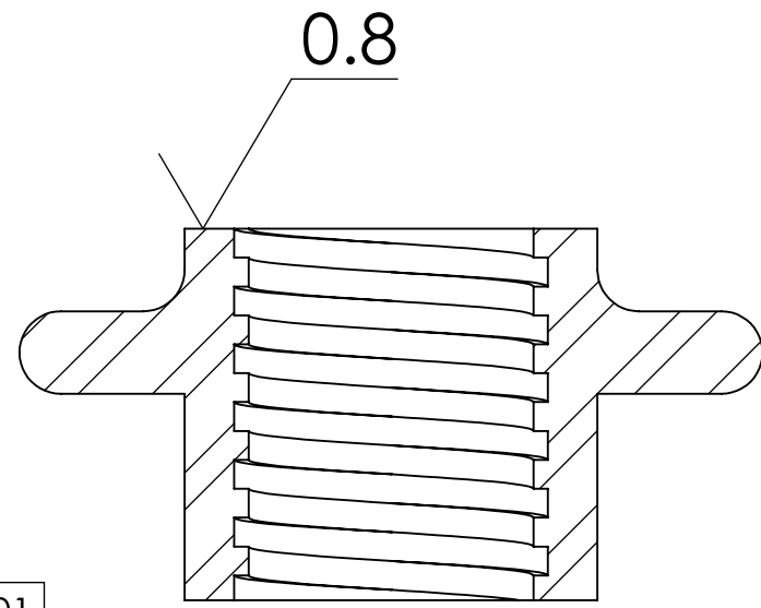
SECTION A-A SCALE 1 : 1 Dia 38 x 7
