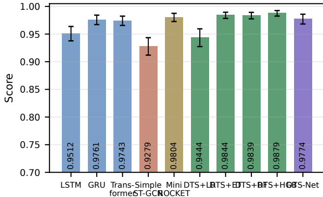
AUROC
