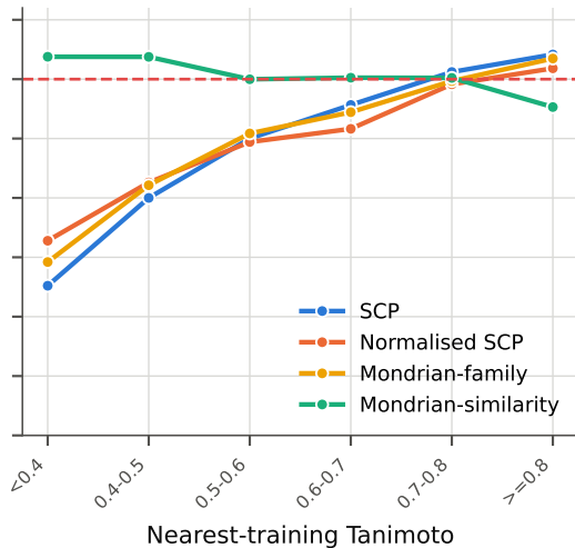
Scaffold
