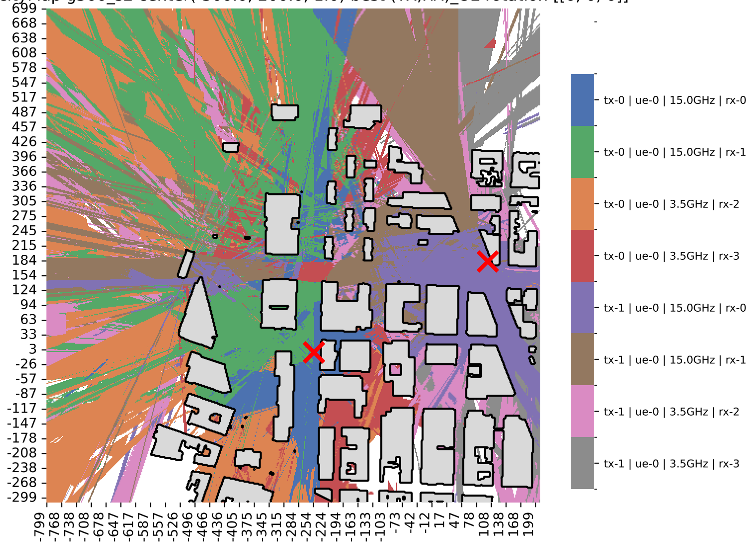
CapacityMap g500_s2 center(-300.0, 200.0, 1.0) best (TX,RX)_UE rotation [[0, 0, 0]]
