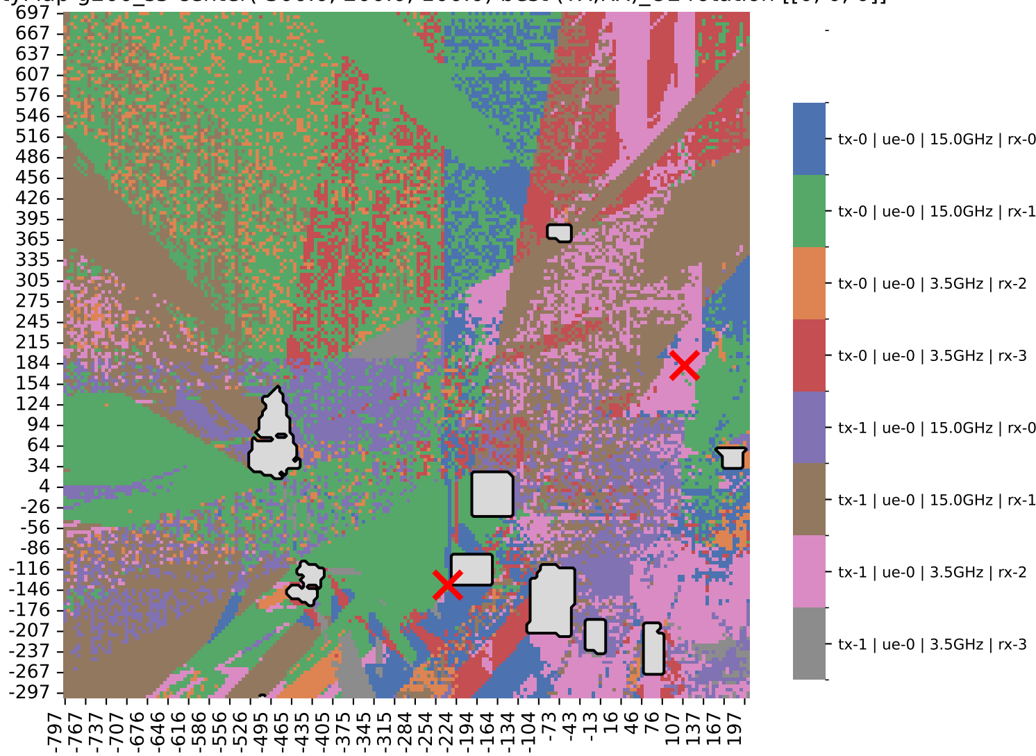
CapacityMap g200_s5 center(-300.0, 200.0, 100.0) best (TX,RX)_UE rotation [[0, 0, 0]]
