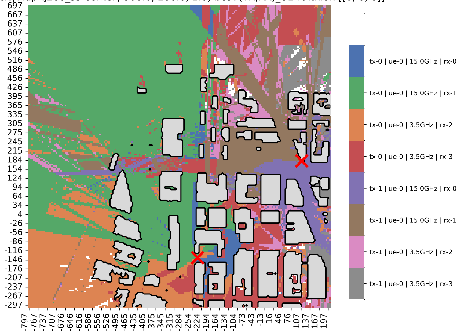
CapacityMap g200_s5 center(-300.0, 200.0, 1.0) best (TX,RX)_UE rotation [[0, 0, 0]]
