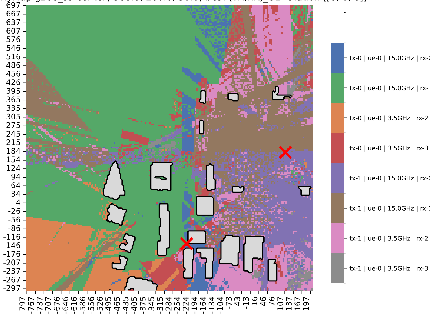
CapacityMap g200_s5 center(-300.0, 200.0, 50.0) best (TX,RX)_UE rotation [[0, 0, 0]]
