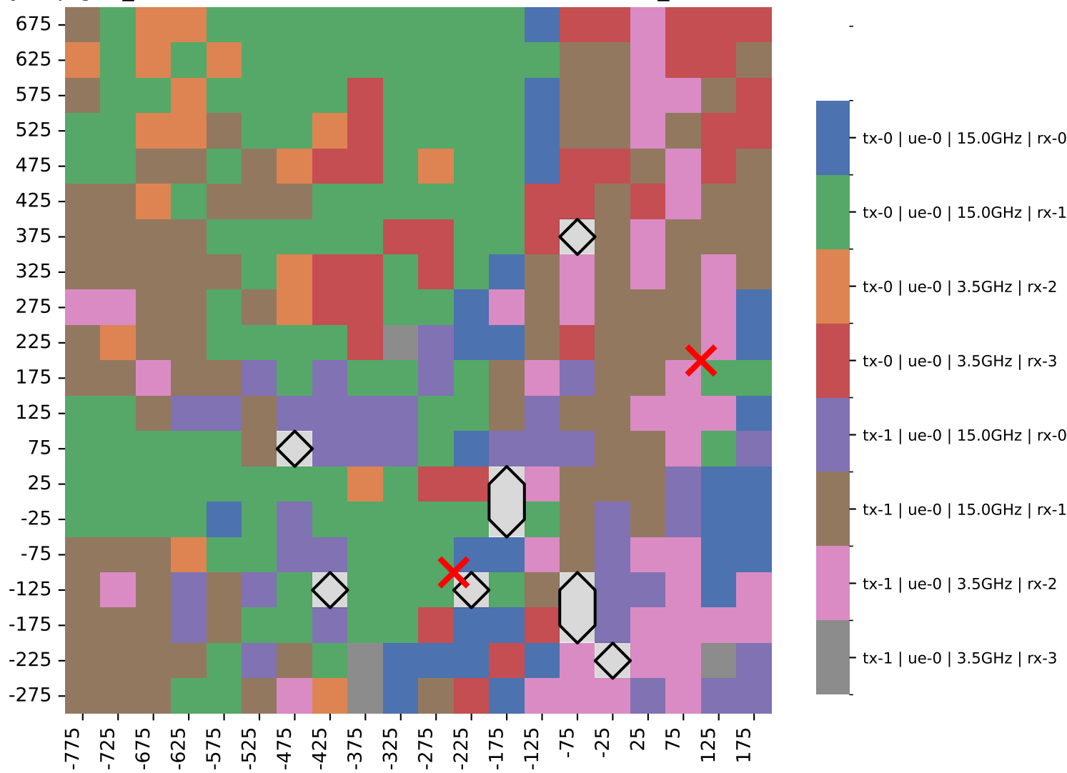
CapacityMap g20_s50 center(-300.0, 200.0, 100.0) best (TX,RX)_UE rotation [[0, 0, 0]]
