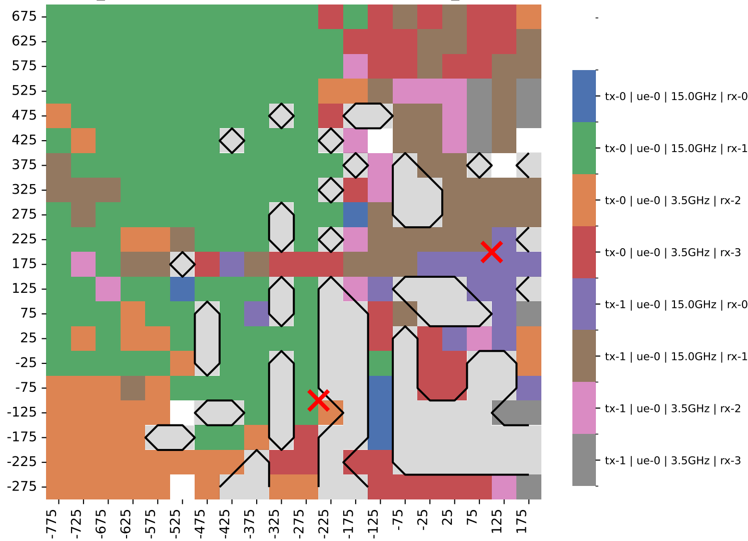
CapacityMap g20_s50 center(-300.0, 200.0, 1.0) best (TX,RX)_UE rotation [[0, 0, 0]]
