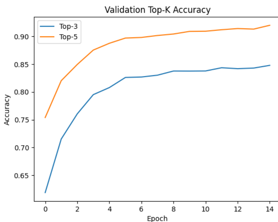
Figura 10: Curvas de precisión top-k del primer modelo con 100k de datos de entrenamiento.
