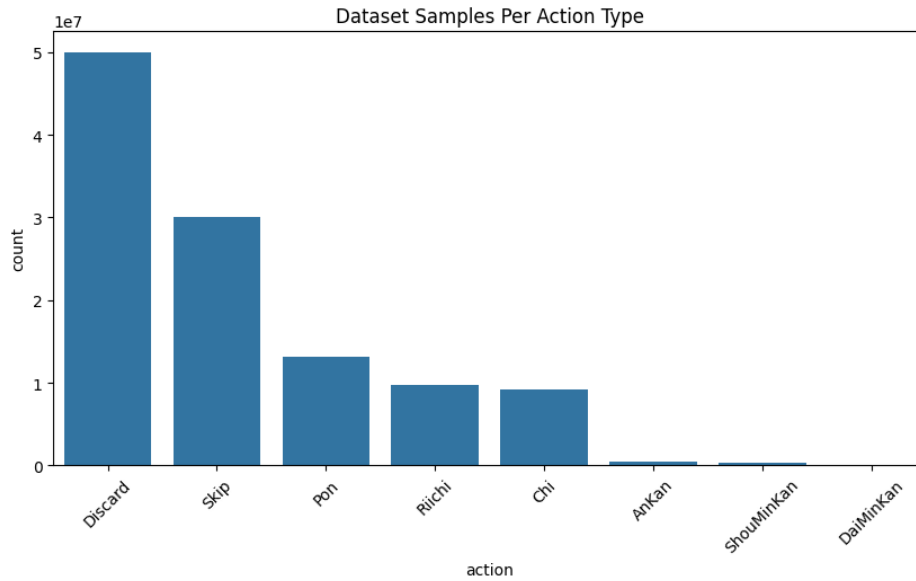
Figura 4: Distribución de Acciones Válidas
