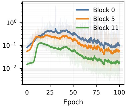
MLP fc2 LoRA-B gradient
