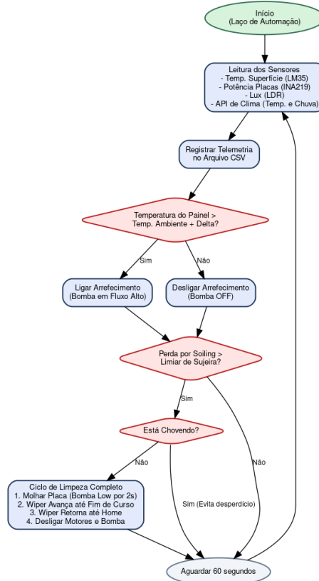
Figura 4: Fluxograma do laço de controle de automação e de tomada de decisão do sistema ASCM. Fonte: Elaborado pelos autores.
